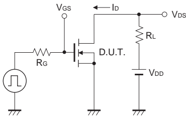
Fig.13 スイッチング時間測定回路
