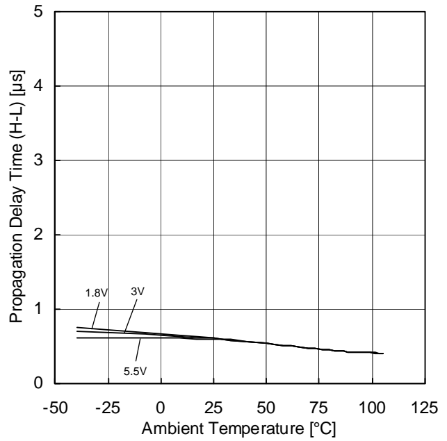
Figure 22. 立ち下がり伝播遅延時間(H-L)－温度特性
