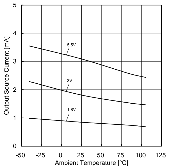
Figure 32. 出力ソース電流－温度特性 (OUT=VDD-0.4V)
