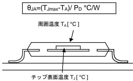
(a) 熱抵抗
