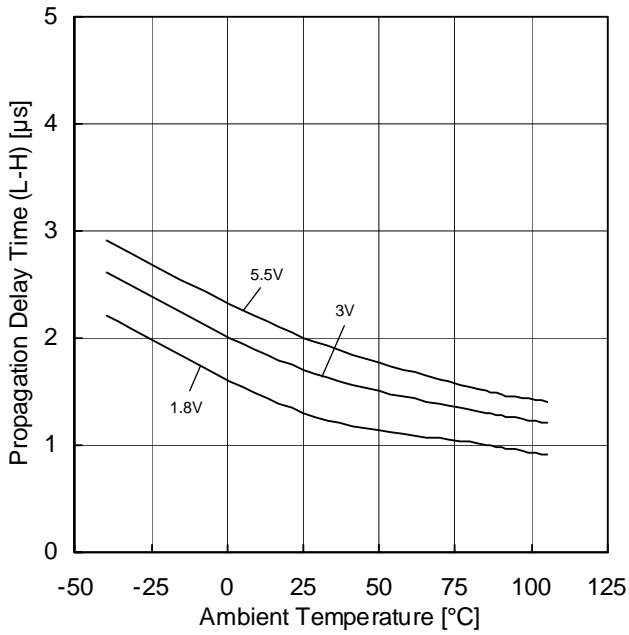
Figure 21. 立ち上がり伝播遅延時間(L-H)－温度特性
