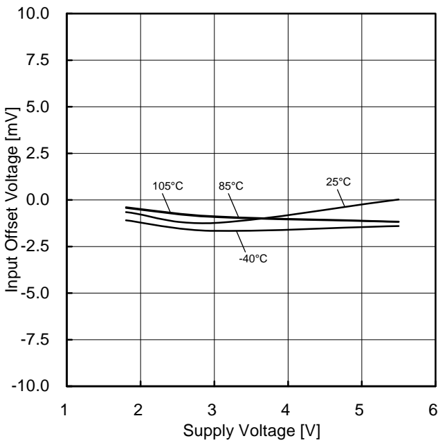
Figure 35. 入力オフセット電圧—電源電圧特性 ( V_{ICM}=V_{DD} , E_K=-V_{DD}/2 )
