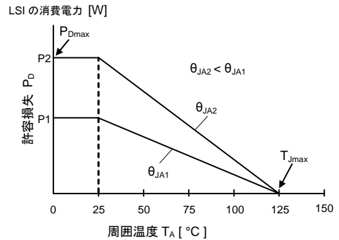
(b) ディレーティング
