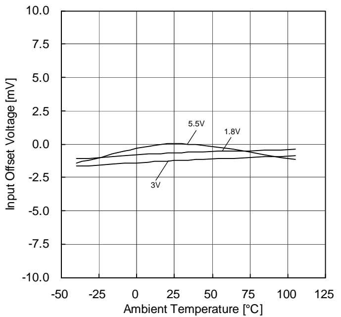
Figure 36. 入力オフセット電圧—温度特性 ( V_{ICM}=V_{DD} , E_K=-V_{DD}/2 )
