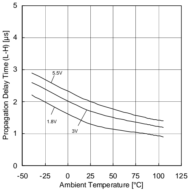
Figure 43. 立ち上がり伝播遅延時間(L-H)－温度特性
