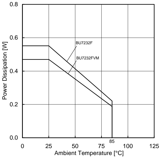
Figure 23. ディレーティングカーブ
