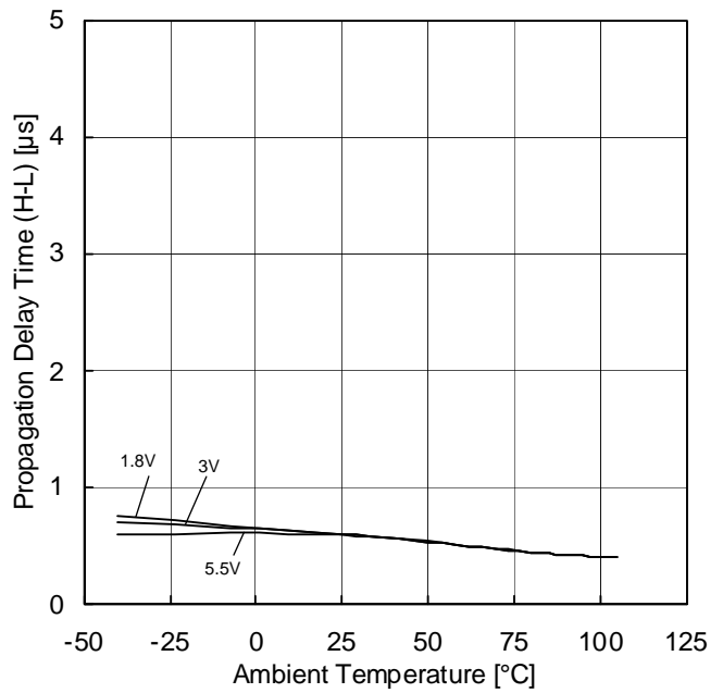
Figure 44. 立ち下がり伝播遅延時間(H-L)－温度特性
