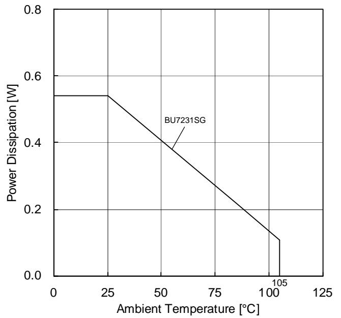
Figure 2. ディレーティングカーブ
