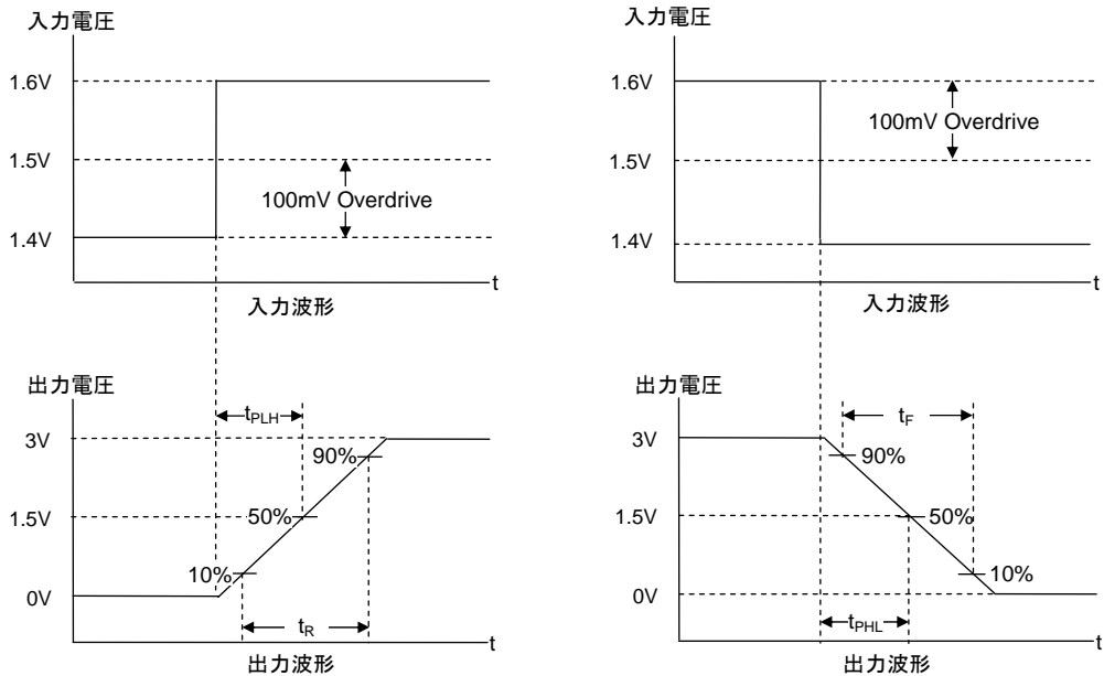
Figure 47. 応答時間測定時 入出力波形
