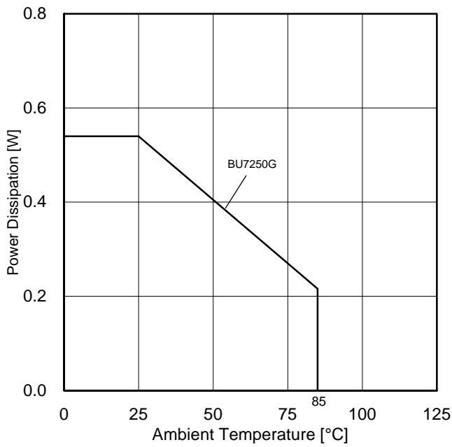
Figure 1. デレーティングカーブ
