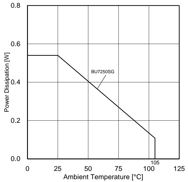
Figure 2. デレーティングカーブ
