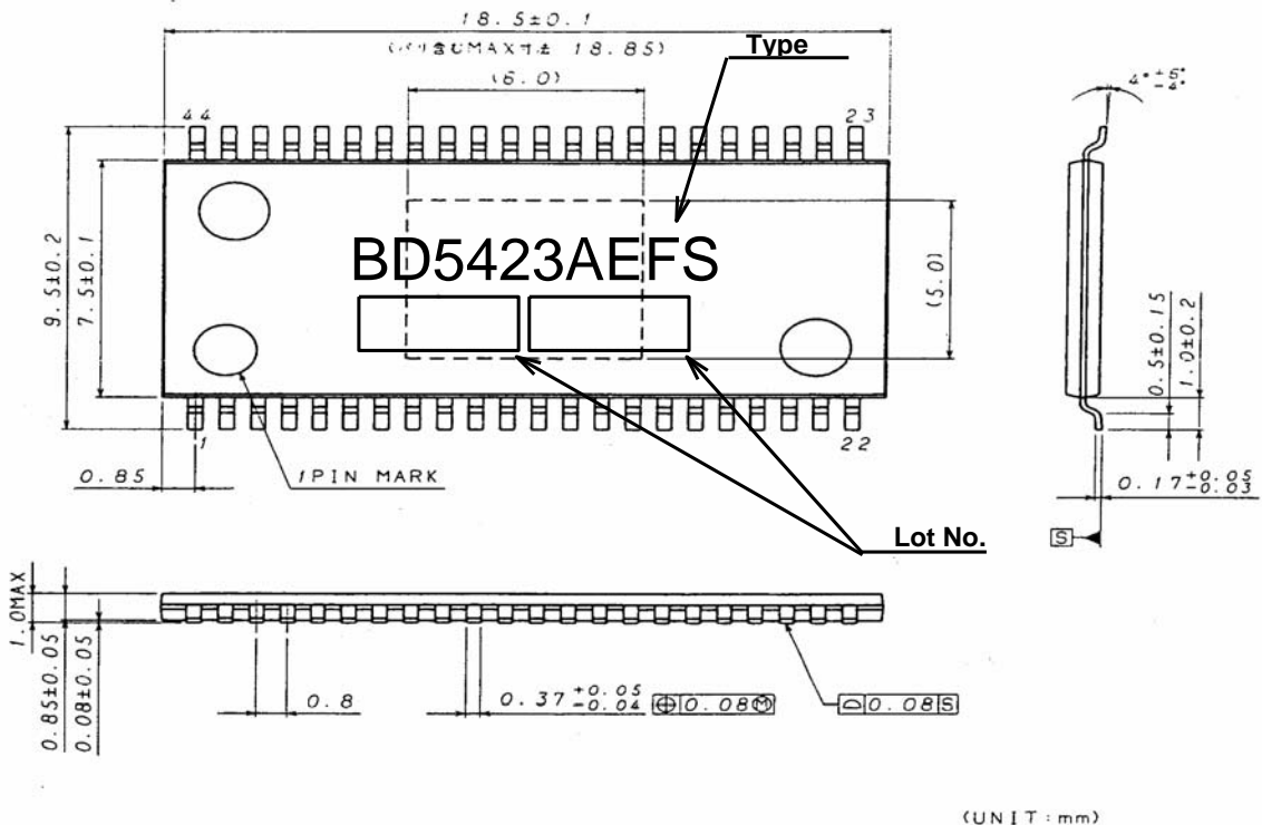
Fig.29 HTSSOP-A44 パッケージ 外形寸法図・標印図
