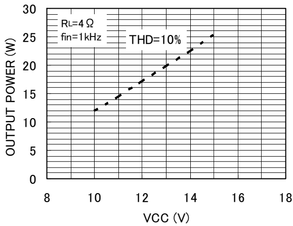
Fig.23 出力電力 - 電源電圧
