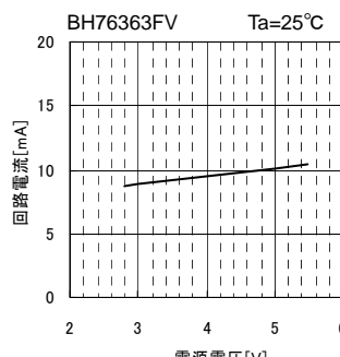
Fig.63 ICC1 vs. 電源電圧
