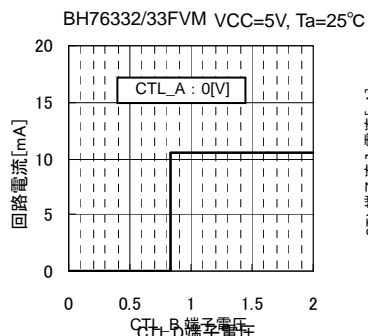
Fig.85 CTL_B 端子電圧 vs 回路電流 (CLT スレッシュホールド)
