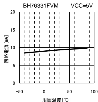
Fig.24 ICC1 vs. 周囲温度
