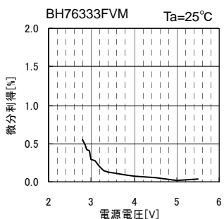
Fig.89 DG vs. 電源電圧
