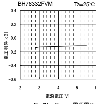
Fig.71 Gv vs. 電源電圧
