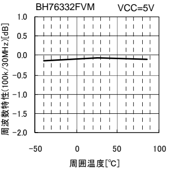
Fig.76 GF vs. 周囲温度
