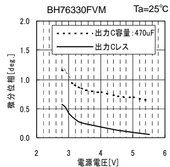
Fig.51 DP vs. 電源電圧
