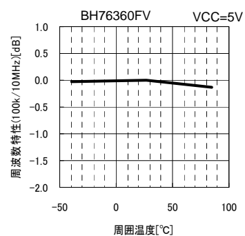
Fig.36 GF vs. 周囲温度
