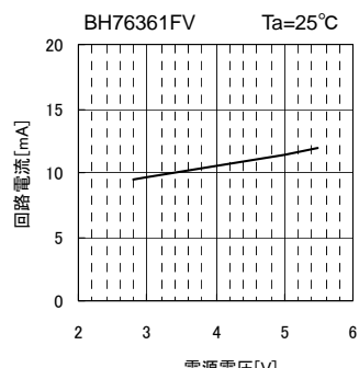
Fig.23 ICC1 vs. 電源電圧
