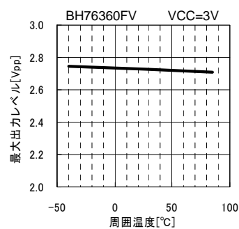
Fig.28 Vom vs. 周囲温度
