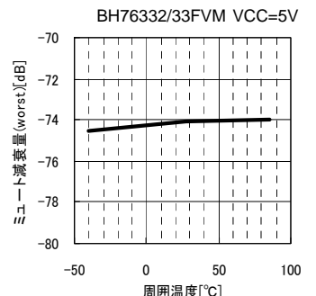
Fig.84 MT(worst) vs. 周囲温度
