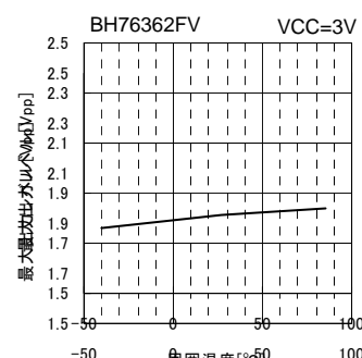
Fig.68 Vom vs. 周囲温度
