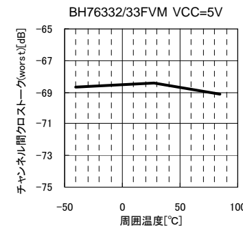
Fig.82 CT(worst) vs. 周囲温度
