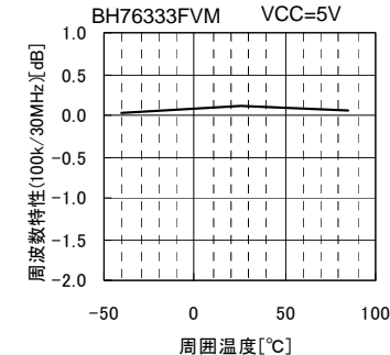
Fig.78 GF vs. 周囲温度
