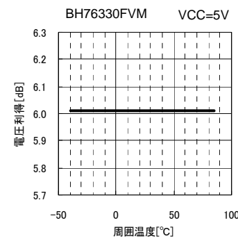
Fig.32 G v vs. 周囲温度
