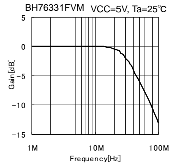
Fig.40 周波数特性
