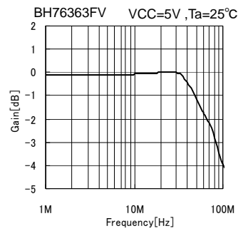
Fig.80 周波数特性
