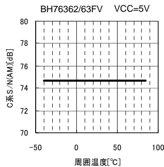
Fig.98 SN_{CA} vs. 周囲温度
