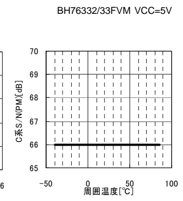
Fig.100 SN_{CP} vs. 周囲温度
