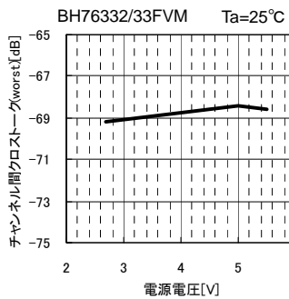
Fig.81 CT(worst) vs. 電源電圧
