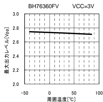
Fig.28 Vom vs. 周囲温度
