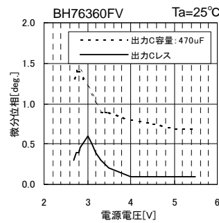
Fig.51 DP vs. 電源電圧
