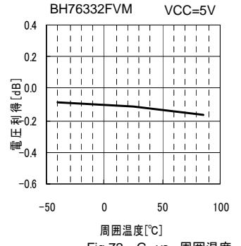
Fig.72 Gv vs. 周囲温度
