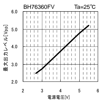
Fig.27 Vom vs. 電源電圧
