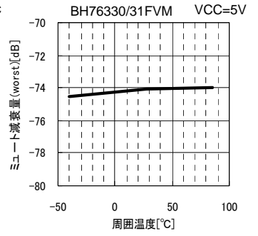
Fig.44 MT(worst) vs. 周囲温度
