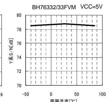
Fig.96 SN_V vs. 周囲温度
