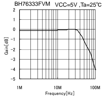
Fig.80 周波数特性
