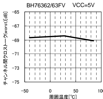
Fig.82 CT(worst) vs. 周囲温度
