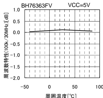
Fig.78 G F vs. 周囲温度
