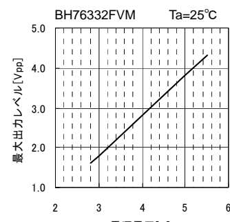
Fig.67 Vom vs. 電源電圧
