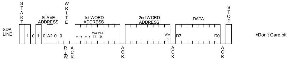
Figure 36. バイトライトサイクル
