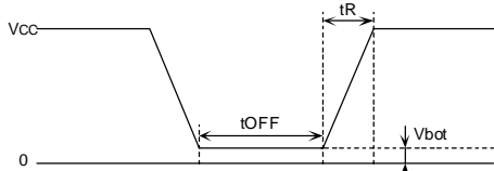
Figure 52. 立ち上がり波形図
