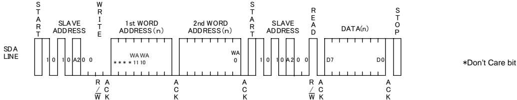
Figure 38. ランダムリードサイクル
