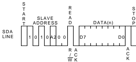
Figure 39. カレントリードサイクル
