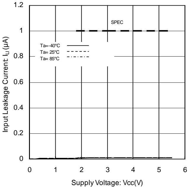
Figure 8. 入力リーク電流 vs 電源電圧 (SCL,WP,A2)
