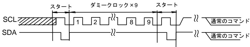
Figure 41.-(b) START+ダミークロック × 9 + START + コマンド入力の場合
