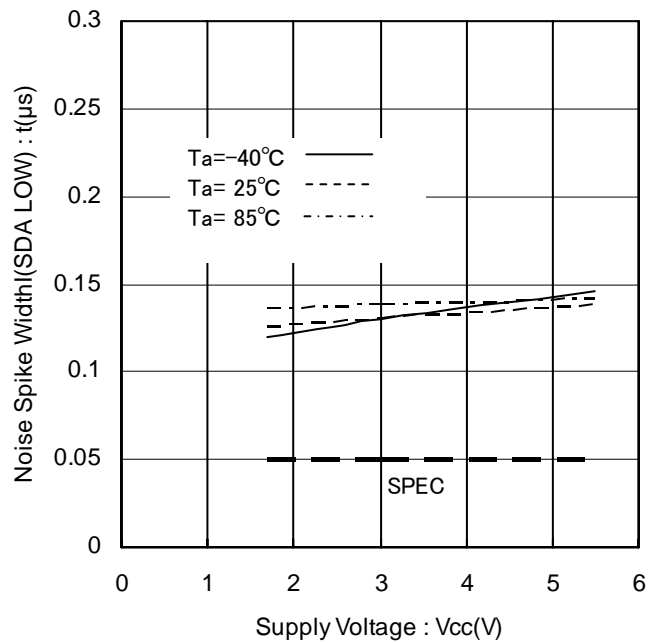
Figure 31. ノイズ除去有効時間 vs 電源電圧 (SDA L)
