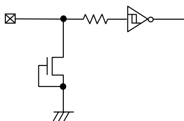
Figure 50. 入力 pin 回路
