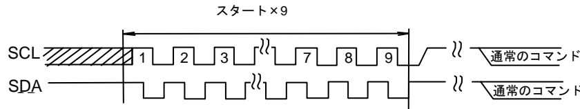
Figure 41.-(c) START × 9 + コマンド入力の場合
