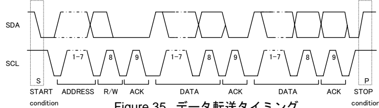
Figure 35. データ転送タイミング
