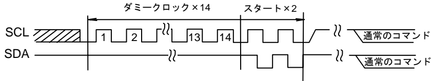
Figure 41.-(a) 14 ダミークロック × 14 + START + START + コマンド入力の場合
