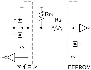
Figure 46. I/O 回路図
