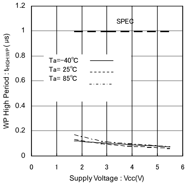
Figure 34. WP 有効時間 vs 電源電圧
