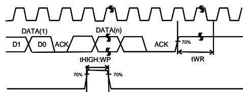
Figure 1.-(e) ライトキャンセル時 WP タイミング
