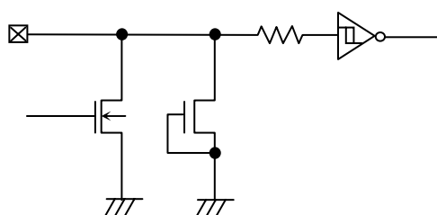
Figure 51. 入出力 pin 回路図
