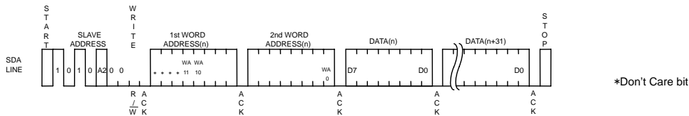
Figure 37. ページライトサイクル
