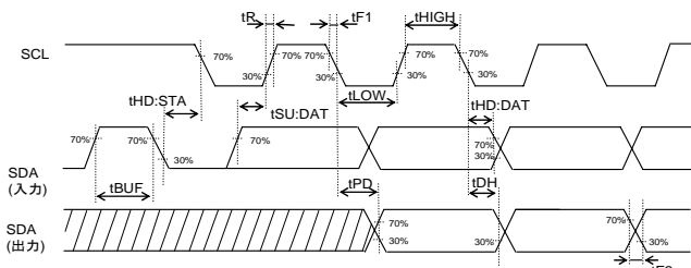
Figure 1.-(a) 同期データ入出力タイミング
