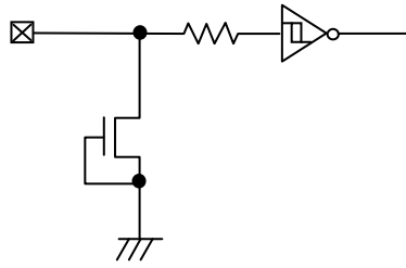
Figure 46. 入力 pin 回路図
