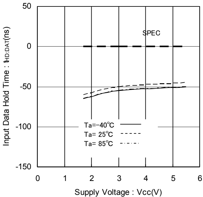
Figure 20. 入力データホールド時間 vs 電源電圧 (LOW)
