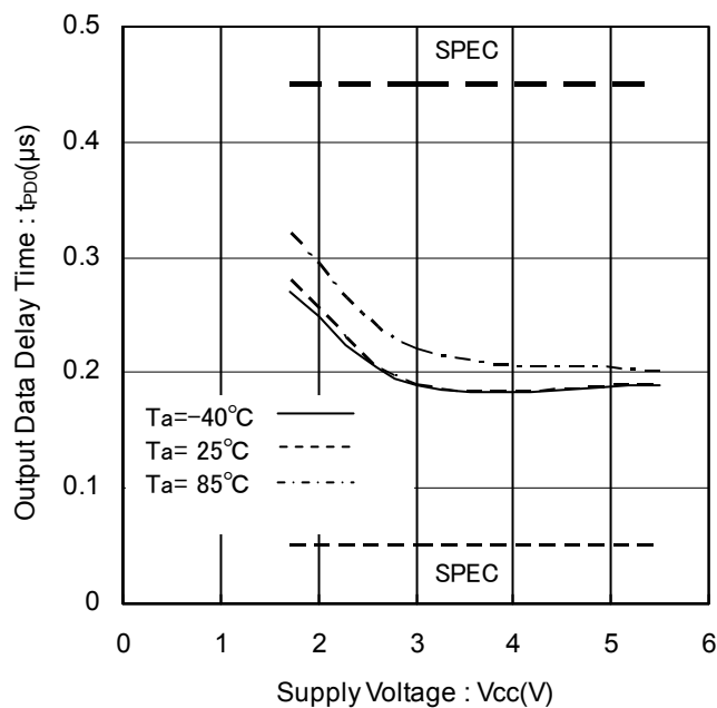
Figure 23. 'L'出力データ遅延時間 vs 電源電圧 (LOW)
