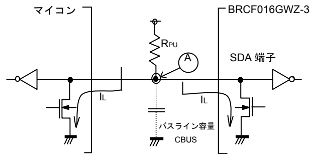
Figure 41. I/O 回路図
