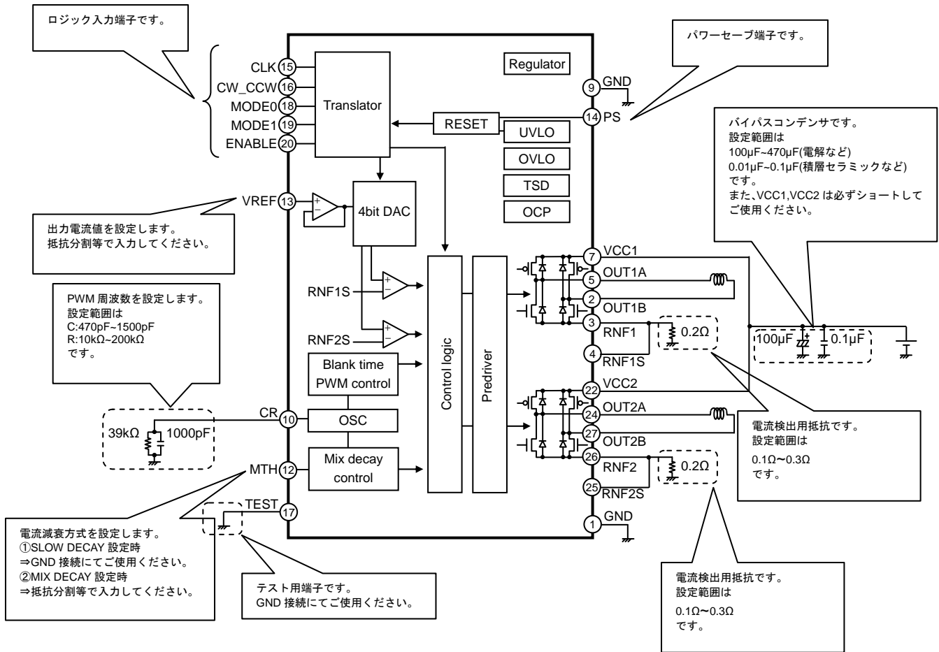
Fig.1 BD63847EFV/BD63843EFV ブロック図・応用回路図
