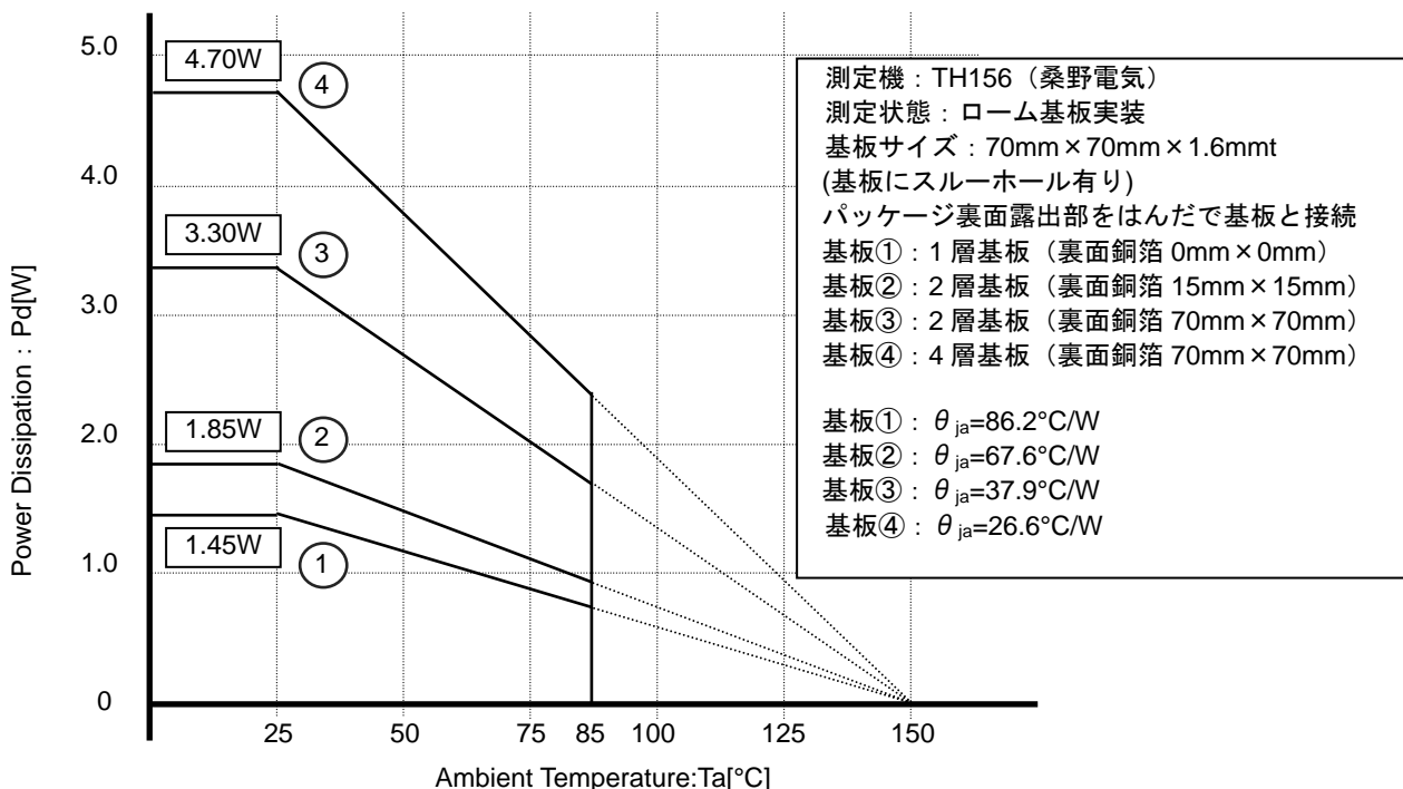
Fig.2 HTSSOP-B28 熱軽減曲線
