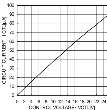
Fig.22 CTL 電圧 vs CTL 電流
