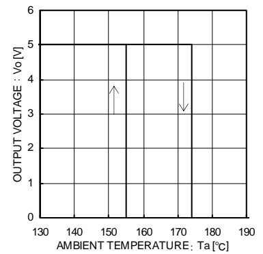
Fig.24 温度保護回路特性
