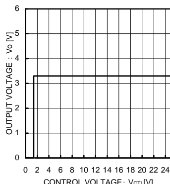
Fig.11 CTL 電圧 vs 出力電圧
