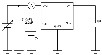
Fig.1 と Fig.13 の測定回路
