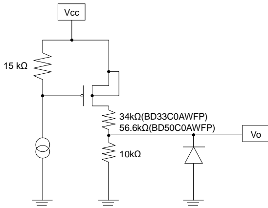
Vo 端子
