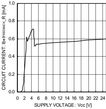
Fig.13 回路電流
