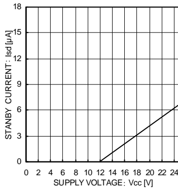
Fig.2 スタンバイ電流
