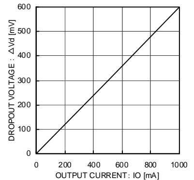
Fig.18 入出力電圧差 (Vcc=Vo × 0.95V) (Io=0mA→1000mA)
