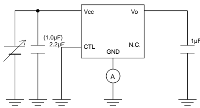
Fig.2 と Fig.14 の測定回路
