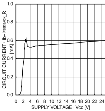
Fig.1 回路電流
