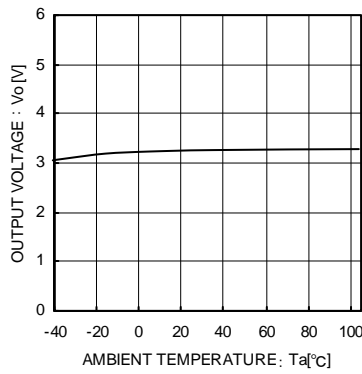
Fig.8 出力電圧温度特性
