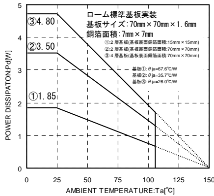
Fig.27(参考データ)
