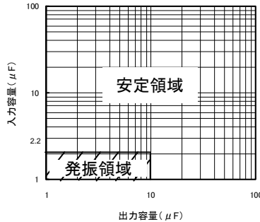
入力容量 vs 出力容量 (参考データ)
