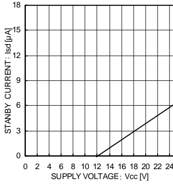
Fig.14 スタンバイ電流
