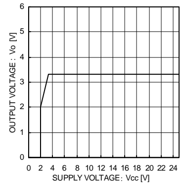
Fig.3 入力安定度 ( I_o=0\text{mA} )
