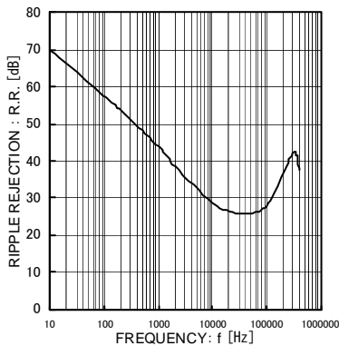
Fig.7 リップルリジェクション ( I_o=100\text{mA} )
