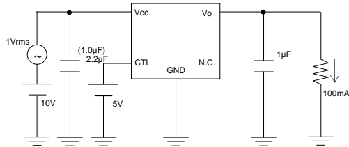
Fig.7 と Fig.19 の測定回路
