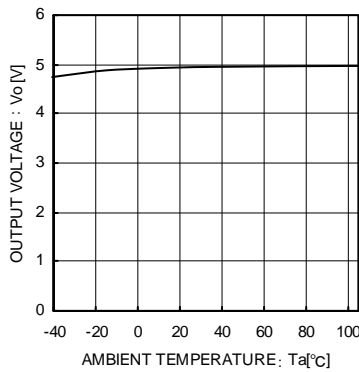
Fig.20 出力電圧温度特性
