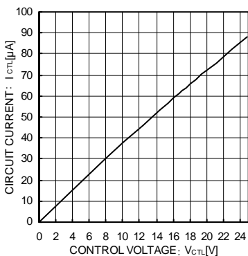
Fig.10 CTL 電圧 vs CTL 電流
