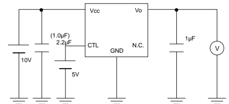
Fig.12 と Fig.24 の測定回路
