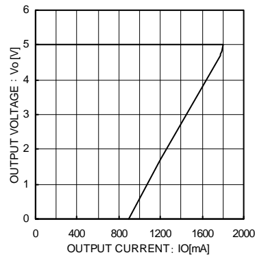
Fig.17 負荷安定度
