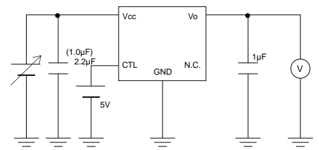
Fig.3 と Fig.15 の測定回路
