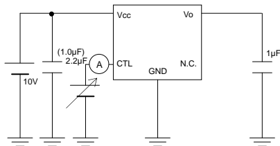
Fig.10 と Fig.22 の測定回路
