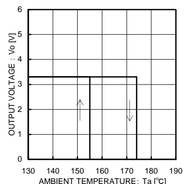
Fig.12 温度保護回路特性
