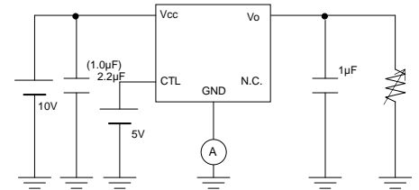
Fig.9 と Fig.21 の測定回路
