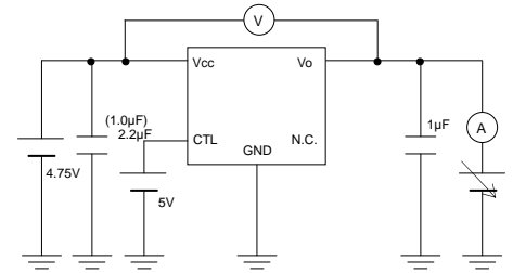
Fig.6 と Fig.18 の測定回路
