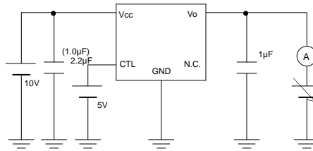
Fig.5 と Fig.17 の測定回路
