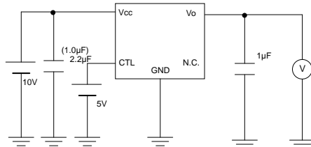
Fig.8 と Fig.20 の測定回路
