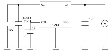
Fig.11 と Fig.23 の測定回路
