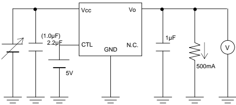
Fig.4 と Fig.16 の測定回路
