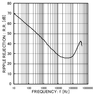
Fig.19 リップルリジェクション (Io=100mA)
