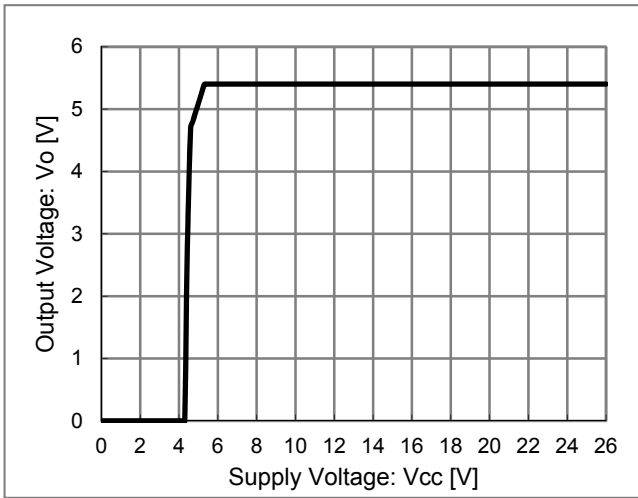
Figure 2. Vcc - Vo
