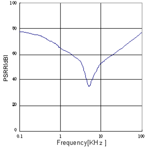
Figure 32. PSRR(Io=0mA)
