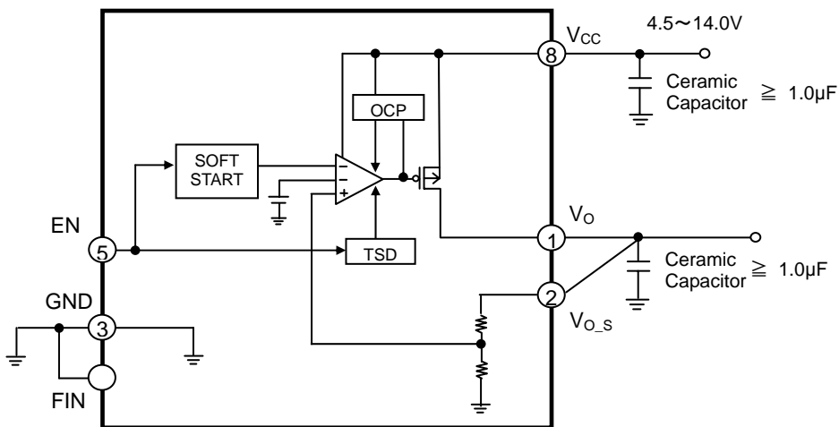
Figure 2. ブロック図 (固定出力タイプ)
