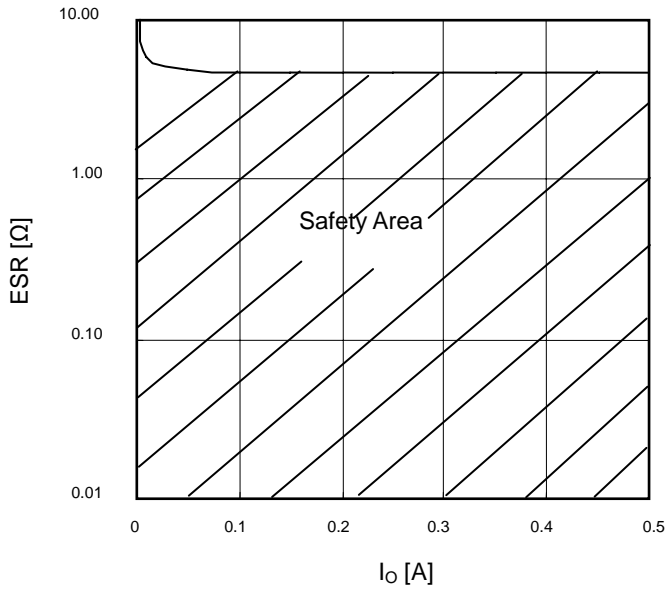
Fig. 31 ESR 安全動作範囲
