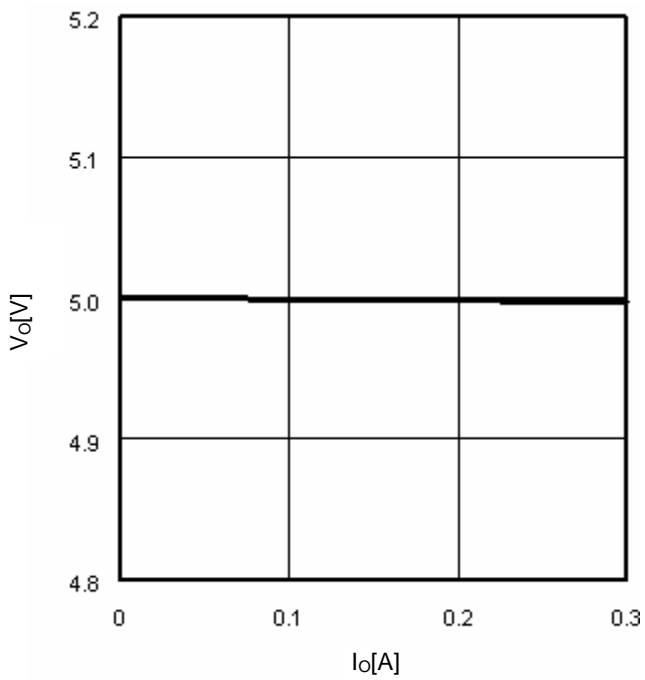
Fig.13 Io-V o
