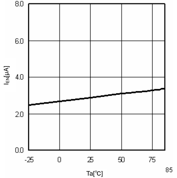
Fig.12 Ta-I EN
