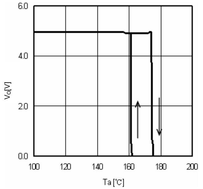
Fig.16 TSD ( I_o=0mA )
