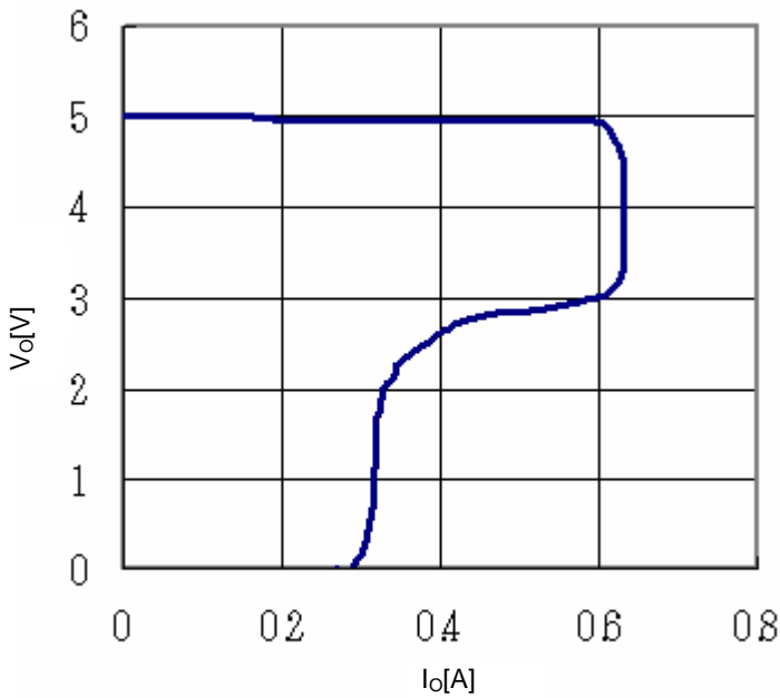
Fig.17 OCP
