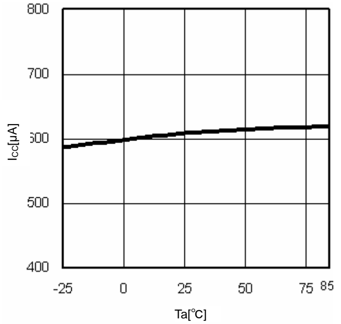
Fig.10 Ta-I CC
