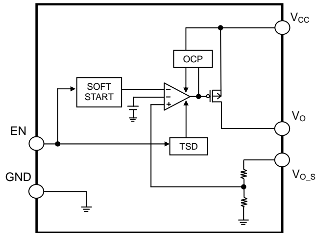
Fig.1 ブロック図
