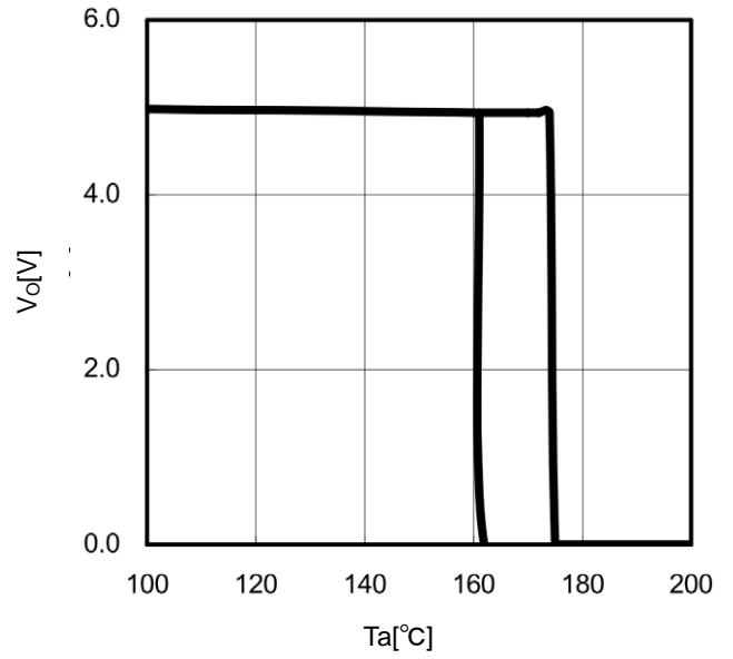
Figure 28. TSD (Io=0mA)
