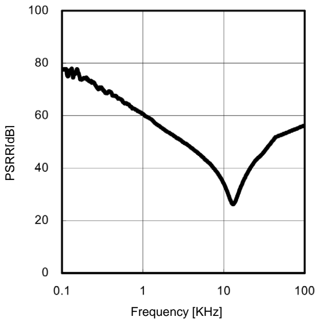
Figure 33. PSRR(I o =0mA)
