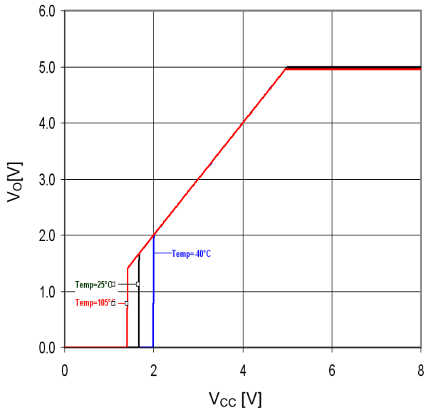
Figure 27. Vcc-Vo (Io=0mA)
