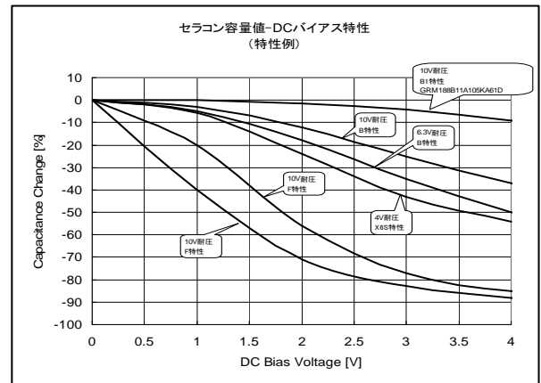
Figure 11. 容量-バイアス特性
