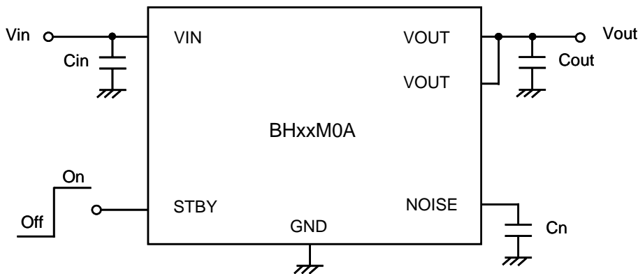
Figure 1. BHxxM0A 基本アプリケーション回路図
