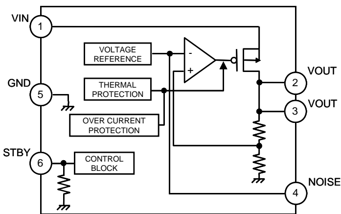
Figure 2. BHxxM0AWHFV ブロック図
