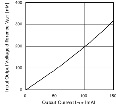
Fig.12 入出力電圧差-出力電流特性 (BH33PB1WHFV)
