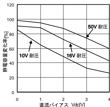
Fig.26 容量-バイアス特性(Y5V)
