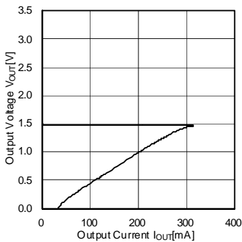
Fig.7 出力電圧-出力電流特性 (BH15RB1WGUT)
