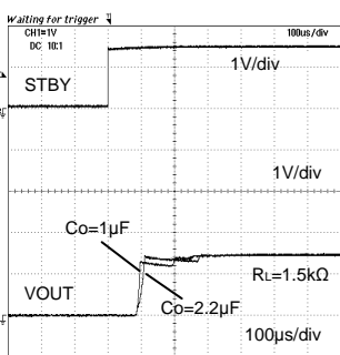
Fig.21 出力電圧立ち上がり時間 (BH15RB1WGUT)
