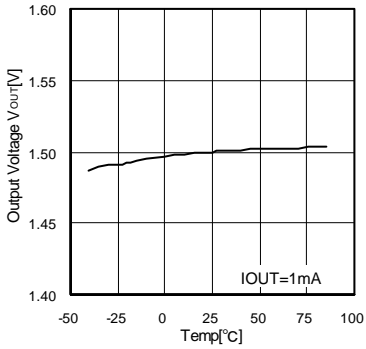
Fig.12 出力電圧-温度特性 (BH15RB1WGUT)
