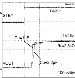
Fig.22 出力電圧立ち上がり時間 (BH28RB1WGUT)
