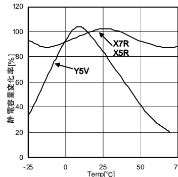
Fig.28 容量-温度特性(X5R,X7R,Y5V)
