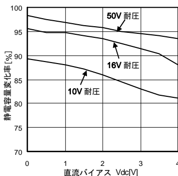
Fig.27 容量-バイアス特性(X5R,X7R)
