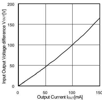
Fig.10 入出力電圧差-出力電流特性 (BH28RB1WGUT)
