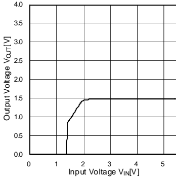
Fig.1 出力電圧-入力電圧特性 (BH15RB1WGUT)
