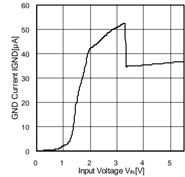
Fig.6 GND 電流-入力電圧特性 (BH33RB1WGUT)
