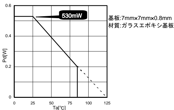
Fig.25 VCSP60N1 許容損失熱軽減特性(参考)
