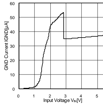
Fig.5 GND 電流-入力電圧特性 (BH28RB1WGUT)
