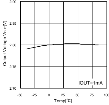
Fig.13 出力電圧-温度特性 (BH28RB1WGUT)
