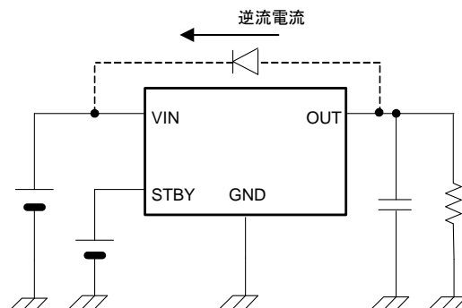
Fig.30 バイパスダイオード接続例
