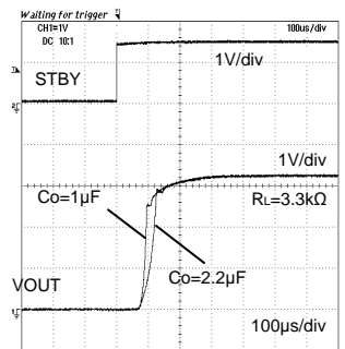
Fig.23 出力電圧立ち上がり時間 (BH33RB1WGUT)
