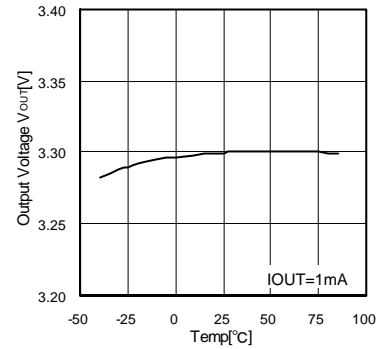
Fig.14 出力電圧-温度特性 (BH33RB1WGUT)
