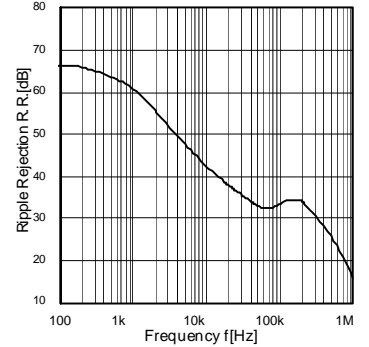
Fig.17 リップルリジェクション (BH33RB1WGUT)
