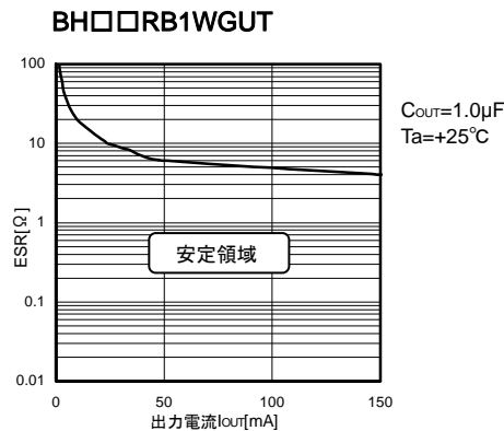
Fig.29 安定動作領域特性(参考)
