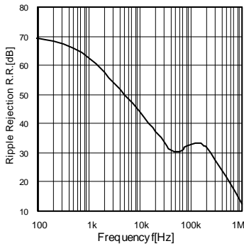
Fig.15 リップルリジェクション (BH15RB1WGUT)
