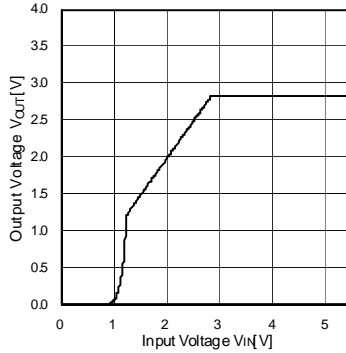
Fig.2 出力電圧-入力電圧特性 (BH28RB1WGUT)
