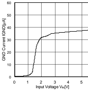
Fig.4 GND 電流-入力電圧特性 (BH15RB1WGUT)
