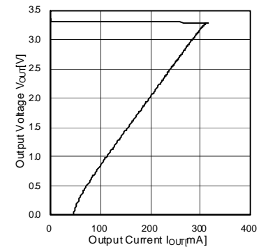
Fig.9 出力電圧-出力電流特性 (BH33RB1WGUT)
