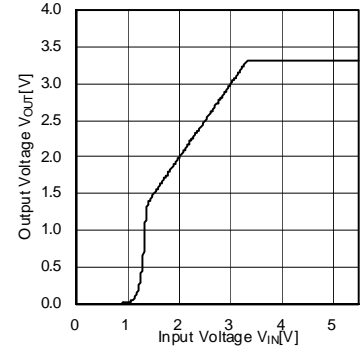
Fig.3 出力電圧-入力電圧特性 (BH33RB1WGUT)
