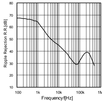
Fig.16 リップルリジェクション (BH28RB1WGUT)
