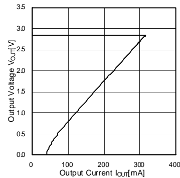
Fig.8 出力電圧-出力電流特性 (BH28RB1WGUT)
