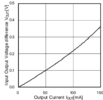
Fig.11 入出力電圧差-出力電流特性 (BH33RB1WGUT)
