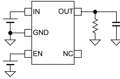
B. EN入力電圧、出力立ち上がり、立ち下がり特性
