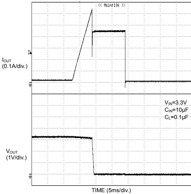
Figure 34. 過電流検出特性 Ramp 出力 (1A/10ms) (BD2202G)
