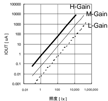
Fig.3 照度 - IOUOUT 特性
