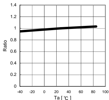
Fig.8 IOUOUT 出力温度特性 (100 lx 時)
