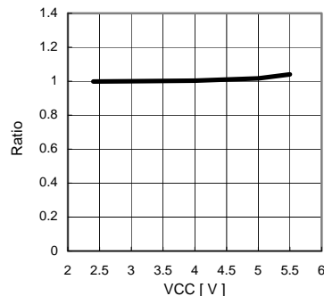
Fig.9 IOUOUT 出力 VCC 依存特性
