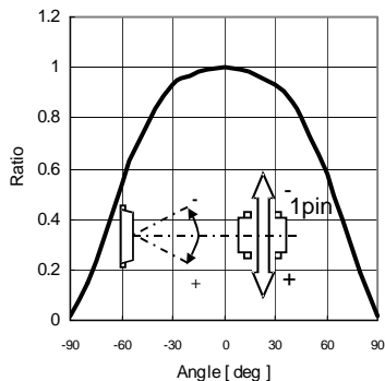
Fig.5 指向角特性 2
