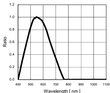
Fig.1 分光感度特性
