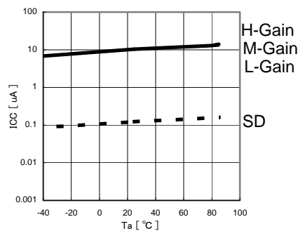
Fig.7 Ta - ICC (0 lx 時)
