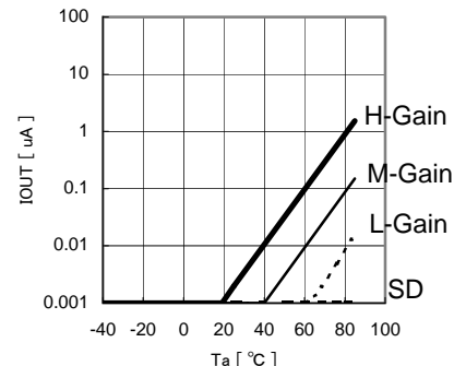
Fig.6 Ta - IOUOUT (0 lx 時)
