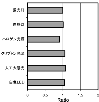
Fig.2 測定結果光源依存 (蛍光灯基準)
