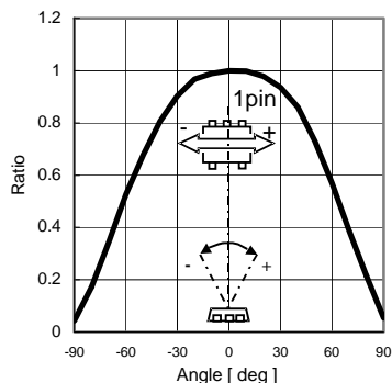
Fig.4 指向角特性 1
