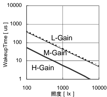
Fig.10 照度 - Wake up Time
